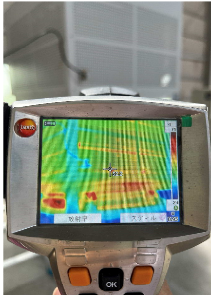
1300°C時表面71°C (Before)
